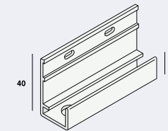
Omrandingsprofiel nr. 2809
