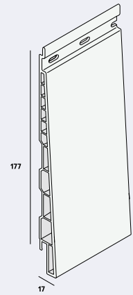
Potdeksel 177 mm nr. 2817
